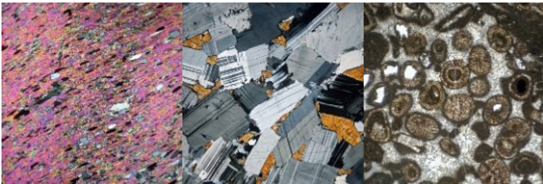
Imágenes al microscopio petroquímico de rocas metamórficas, ígneas y sedimentarias donde se puede observar la distinta composición mineralógica. Biblioteca de imágenes, Department of EarthSciences, Oxford University.
